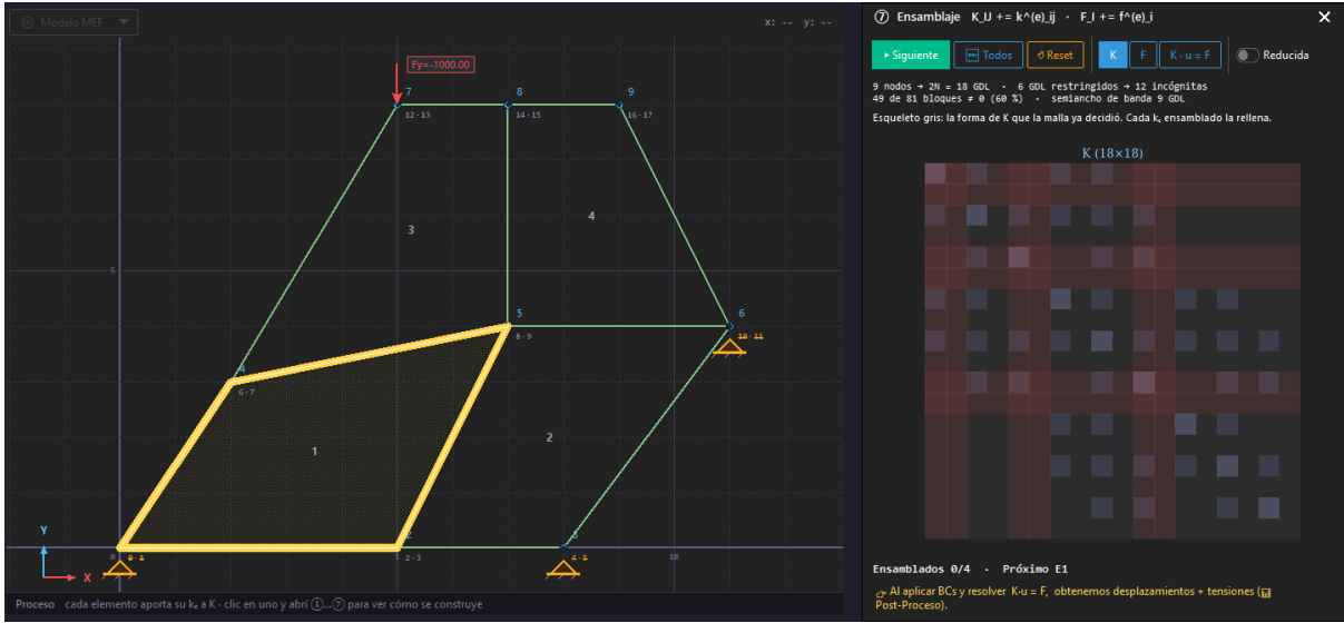
Figura B.13 Módulo M7 (ensamblaje). El aporte de cada matriz elemental k_e a la matriz global K y el patrón de dispersión resultante.
