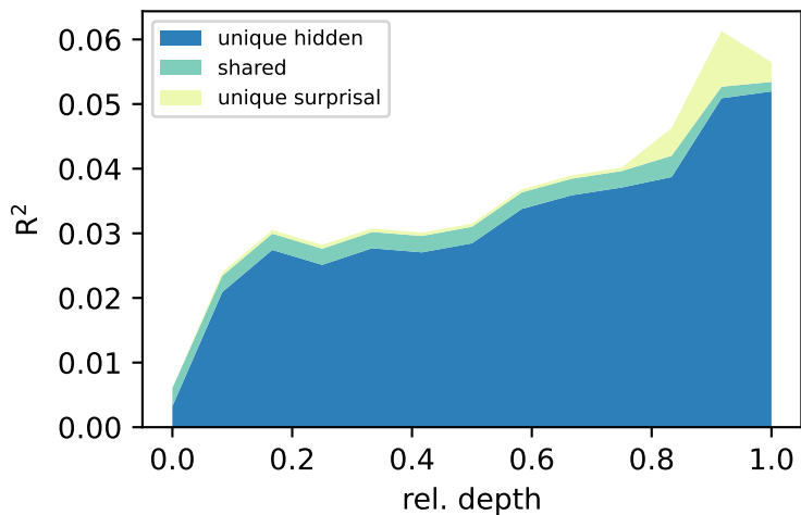
pythia-410m
