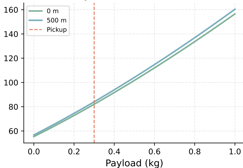
(d) Payload vs Hover Power (W)
