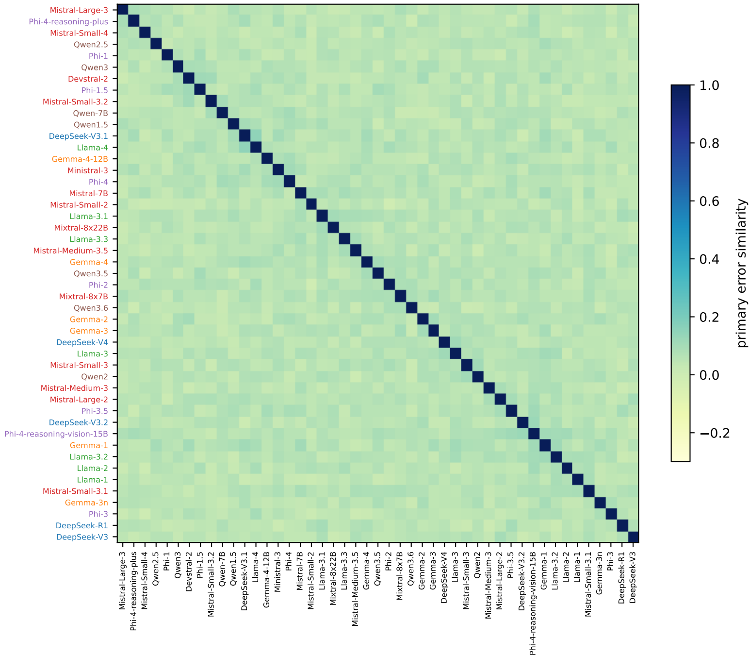
Pairwise error similarity (average-linkage order)
