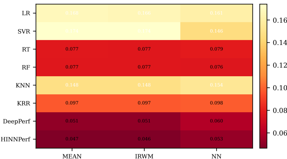
Absolute — MIBRE
