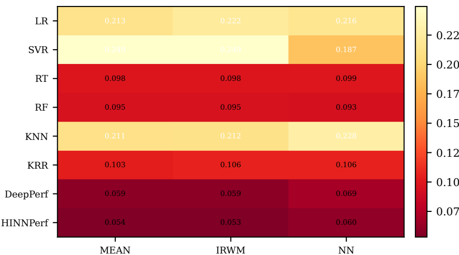
Absolute — MIBRE
