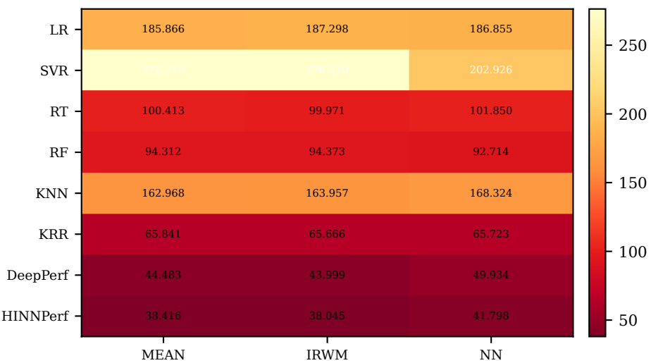
Absolute — MBRE
