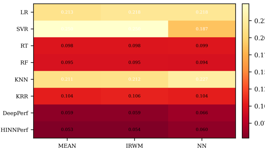
Absolute — MIBRE
