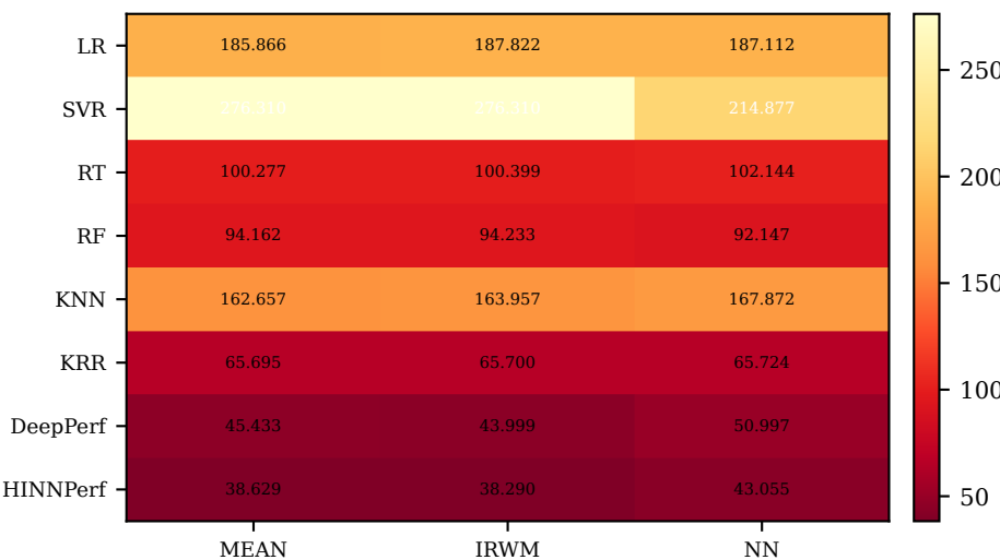
Absolute — MBRE
