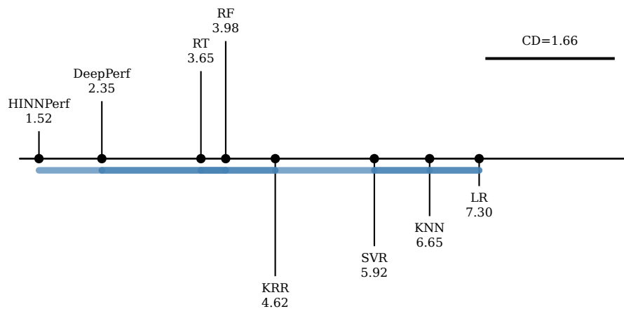
MBRE
