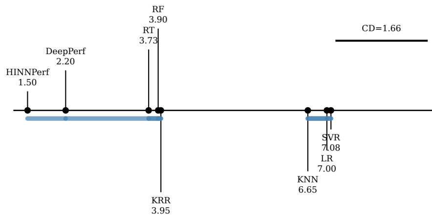
MIBRE
