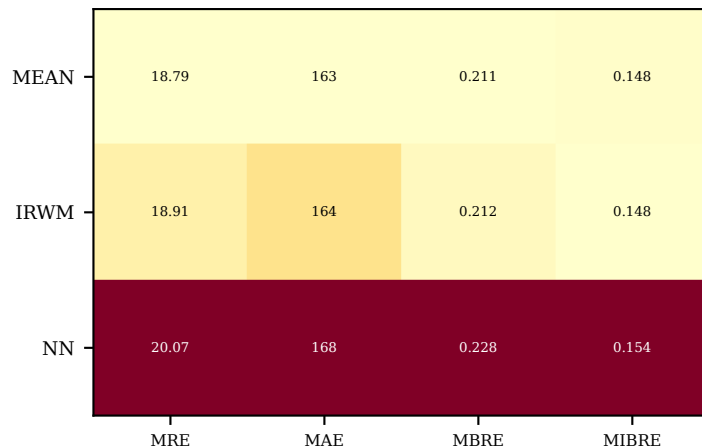
KNN
