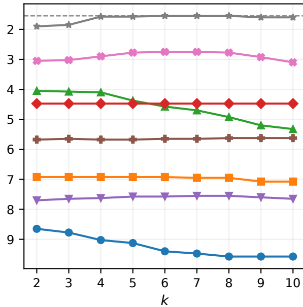
IRWM
