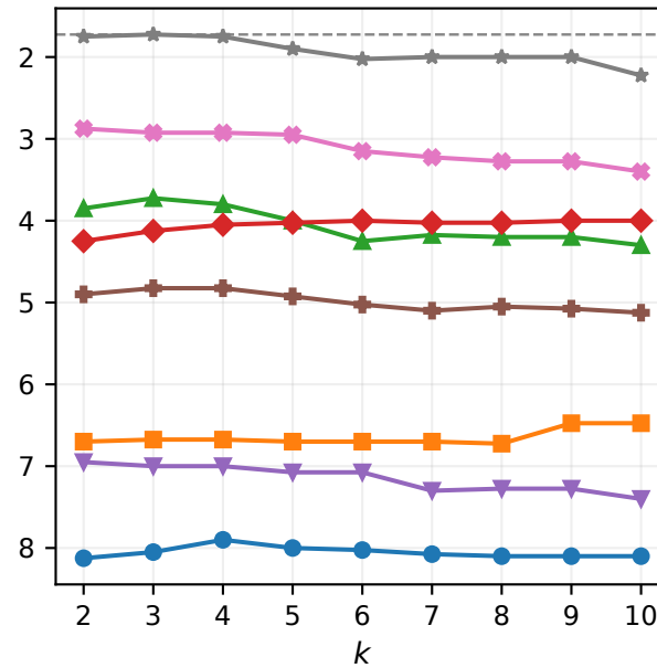
NN
