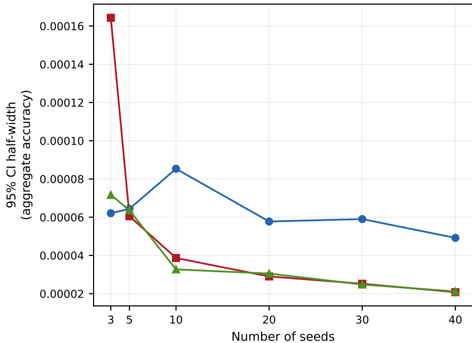
CSE-CIC-IDS2018
