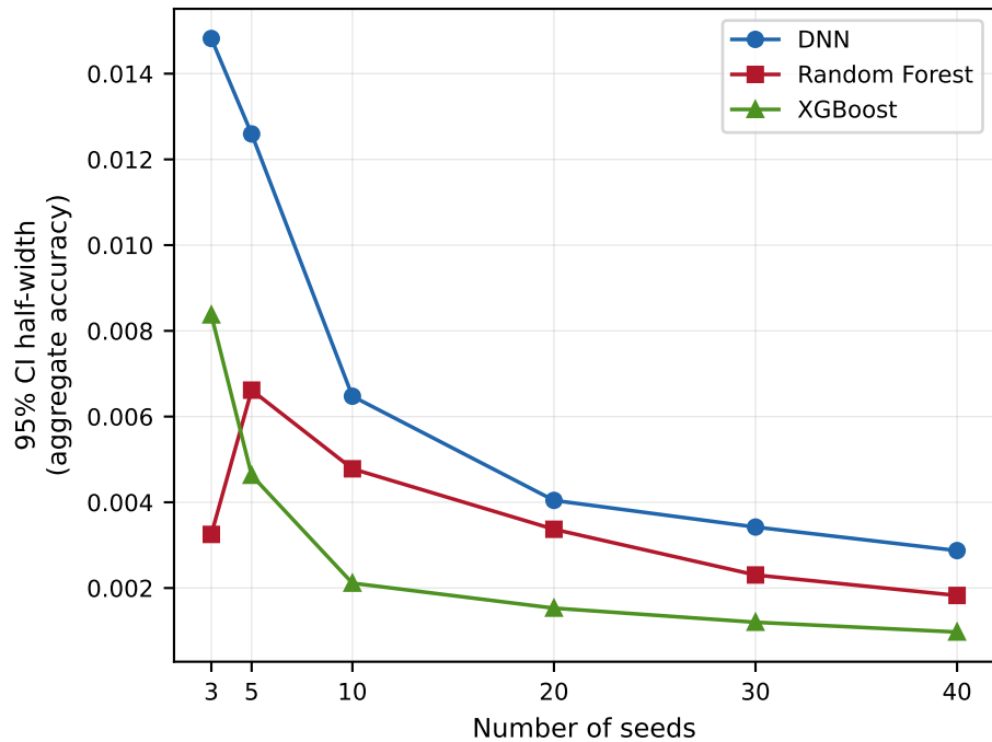
NSL-KDD
