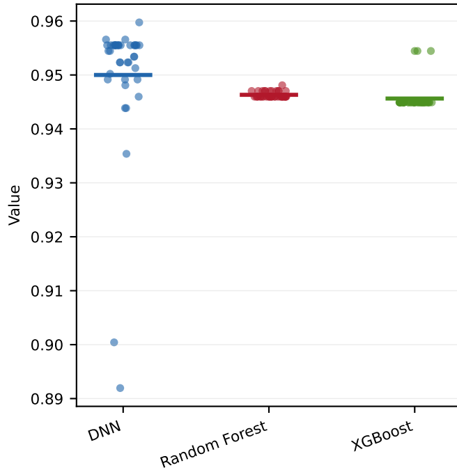
Brute-force recall
