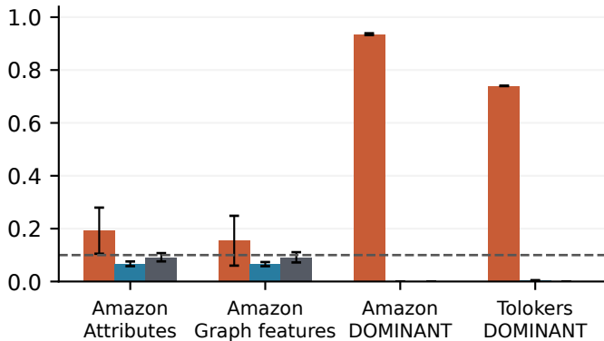
Mean FDP
