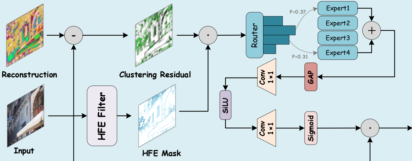
(d) Local High-Frequency Module (LHF)
