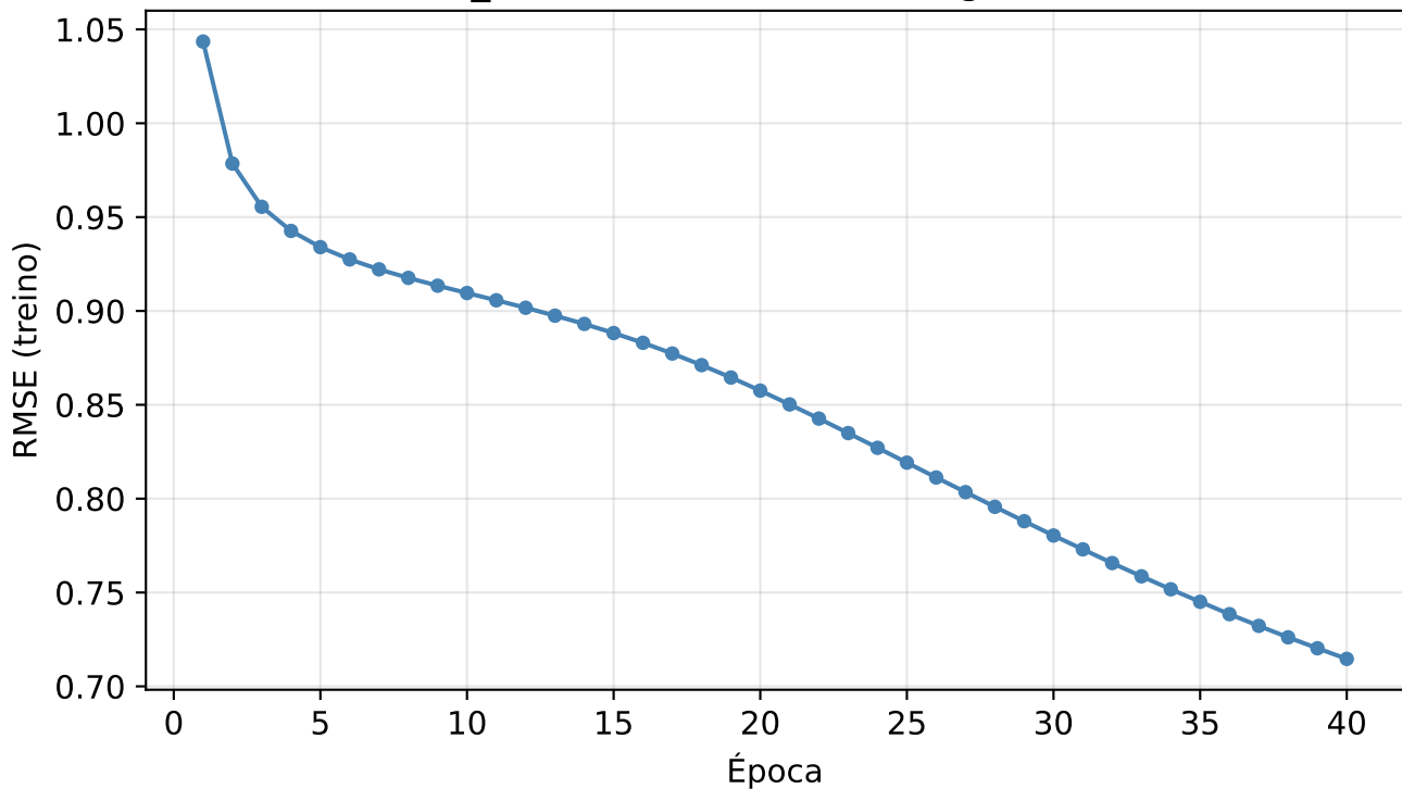
Curva de Convergência do SGD — Regularized SVD (n_factors=20, lr=0.005, reg=0.02)
