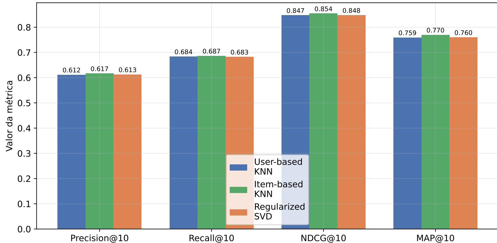
Métricas de Qualidade da Recomendação em K=10 (5-fold CV, relevante = nota real \geq 4 )
