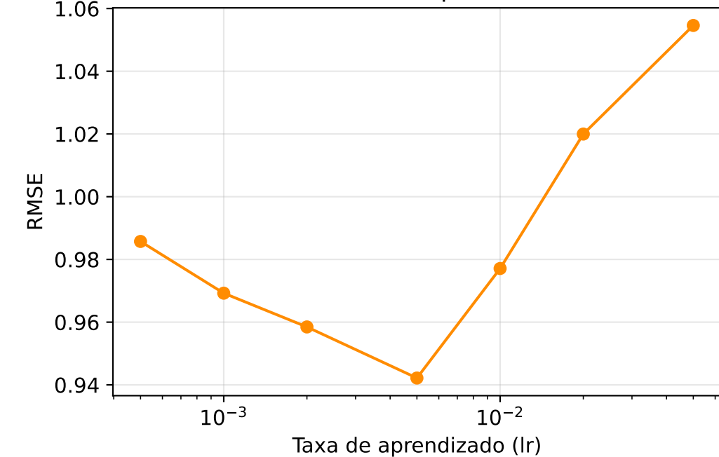
RMSE vs Taxa de aprendizado (lr)
