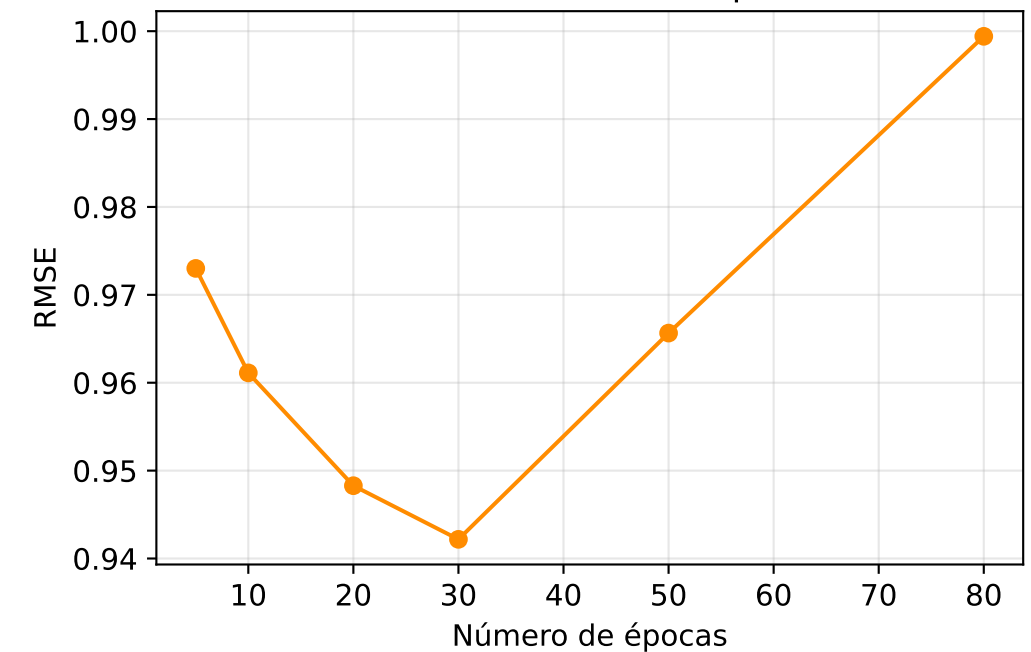
RMSE vs Número de épocas
