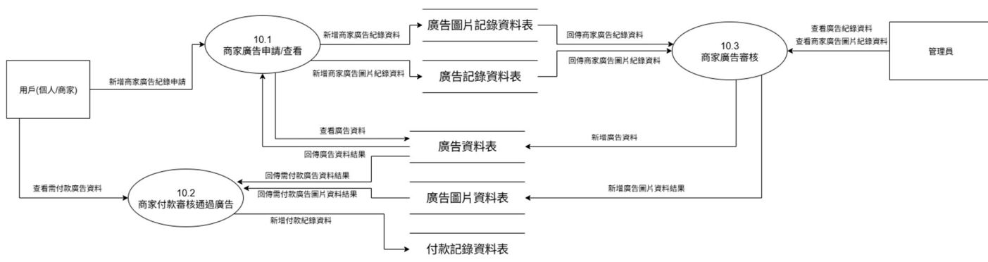
圖 6-1-13 DFD 圖10
