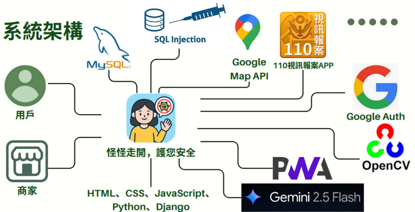
圖 3-1-1 系統架構圖
