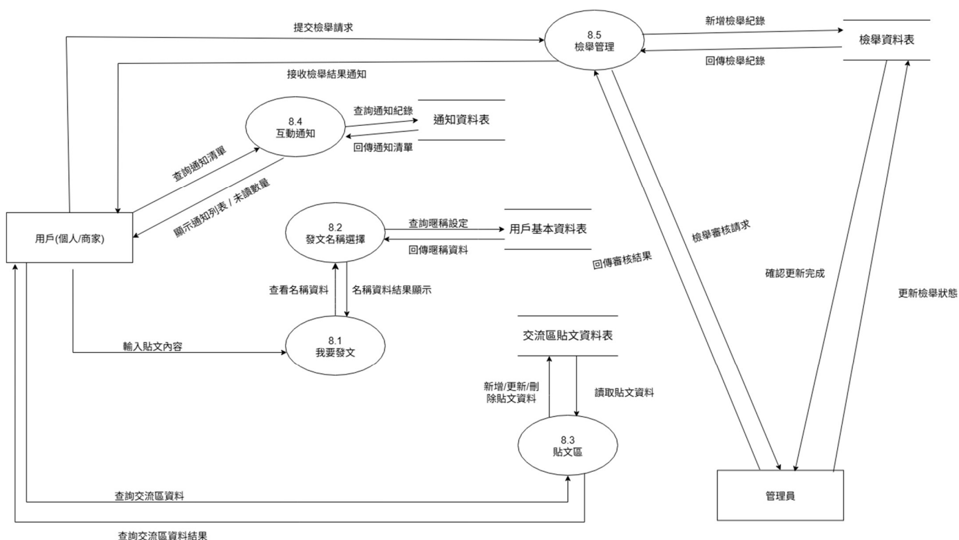
圖 6-1-10 DFD 圖8
