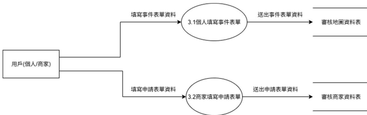
圖 6-1-4 DFD 圖3
