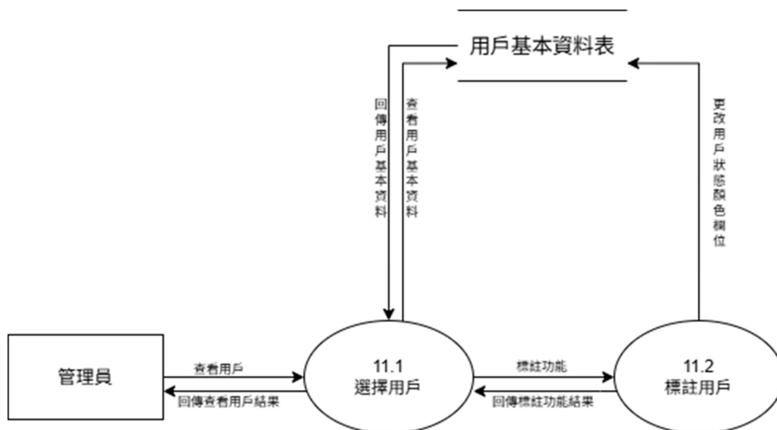
圖 6-1-14 DFD 圖11
