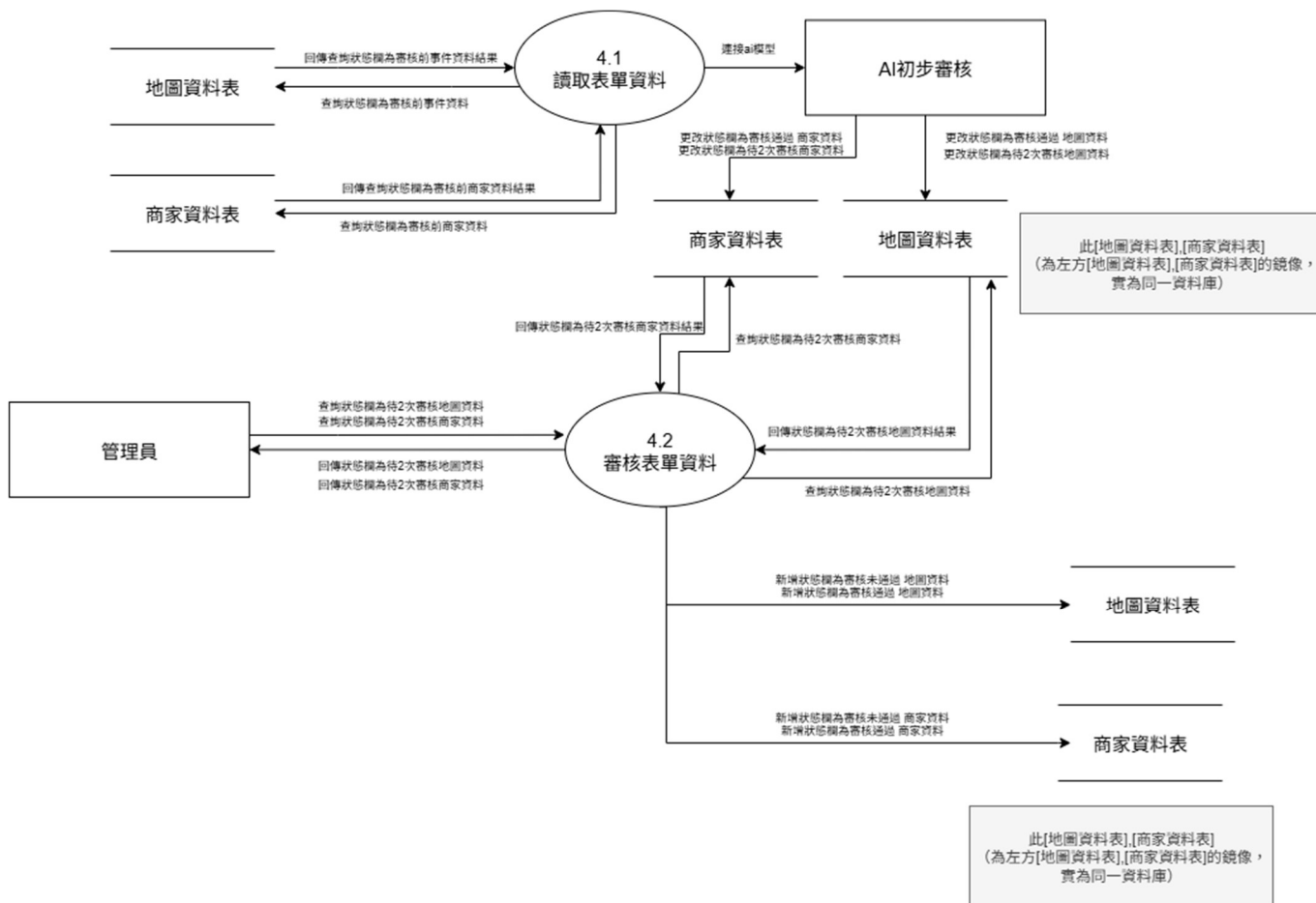
圖 6-1-6 DFD 圖4
