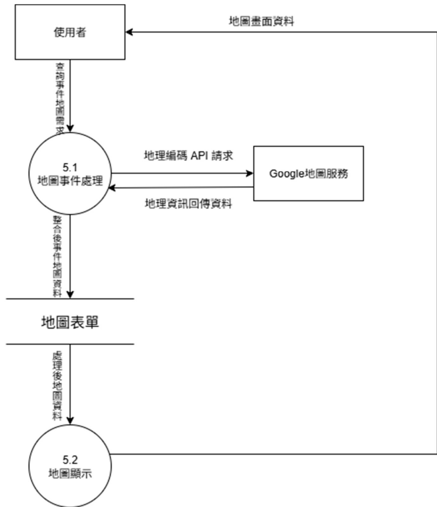
圖 6-1-7 DFD 圖5
