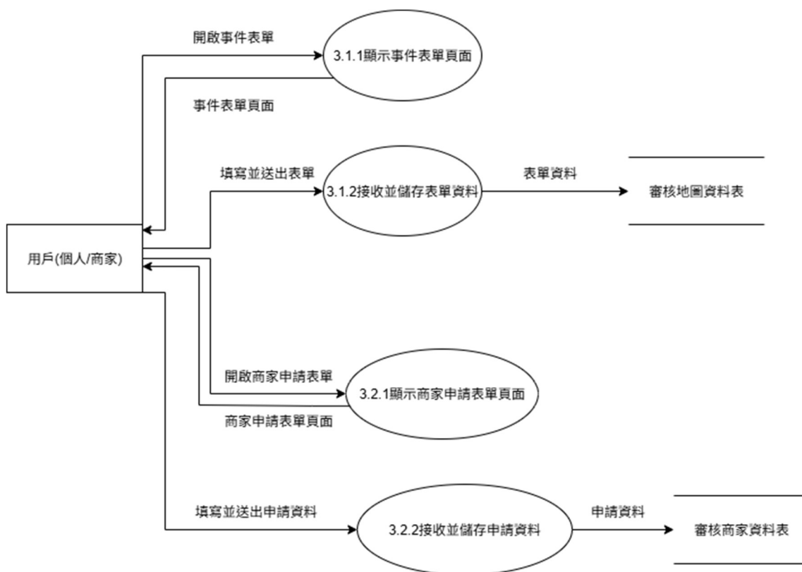
圖 6-1-5 DFD 圖3.1
