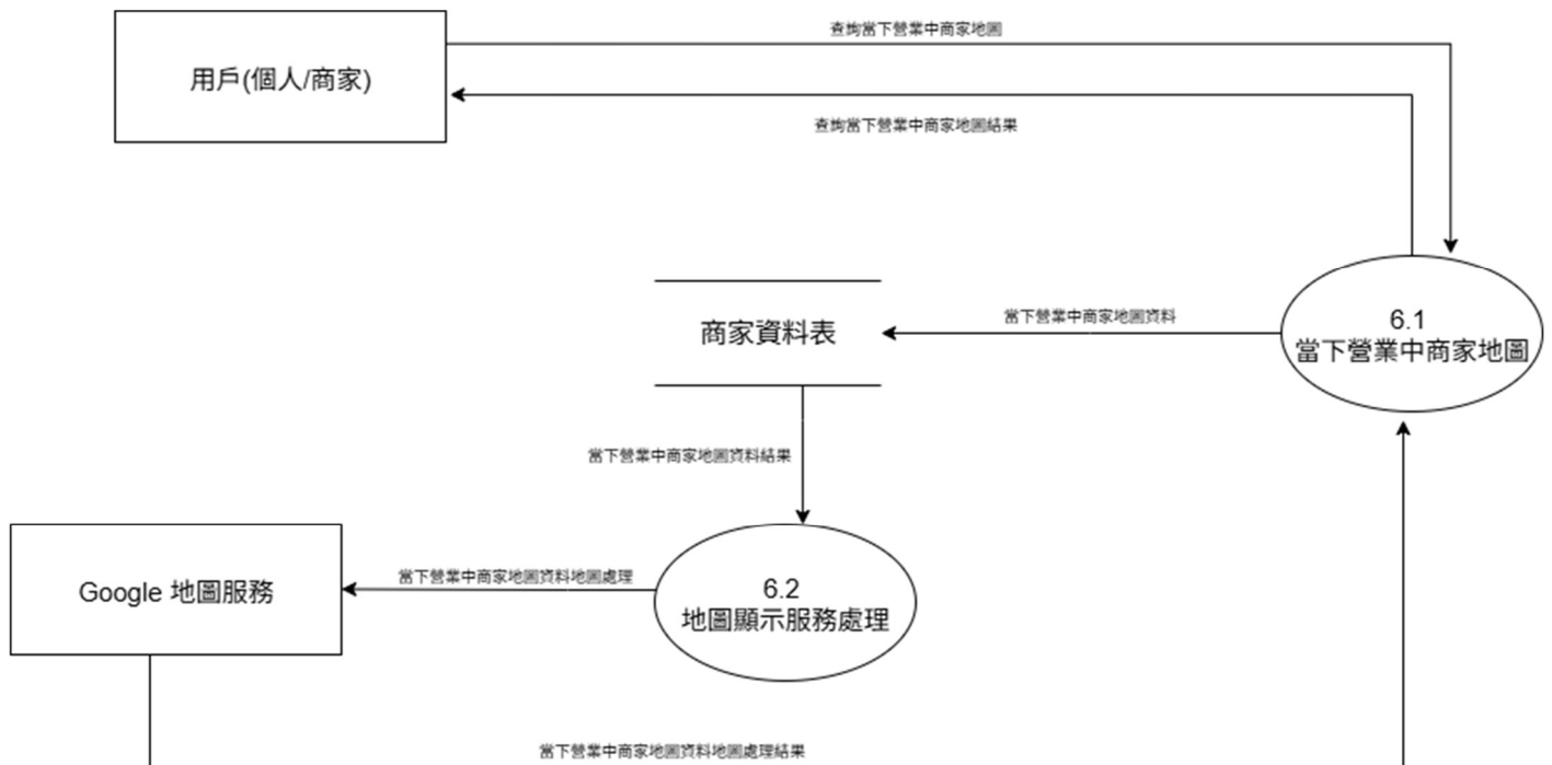
圖 6-1-8 DFD 圖6
