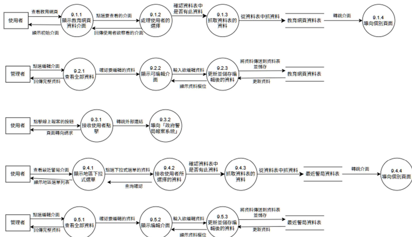
圖 6-1-12 DFD 圖9.1 9.2 9.3 9.4
