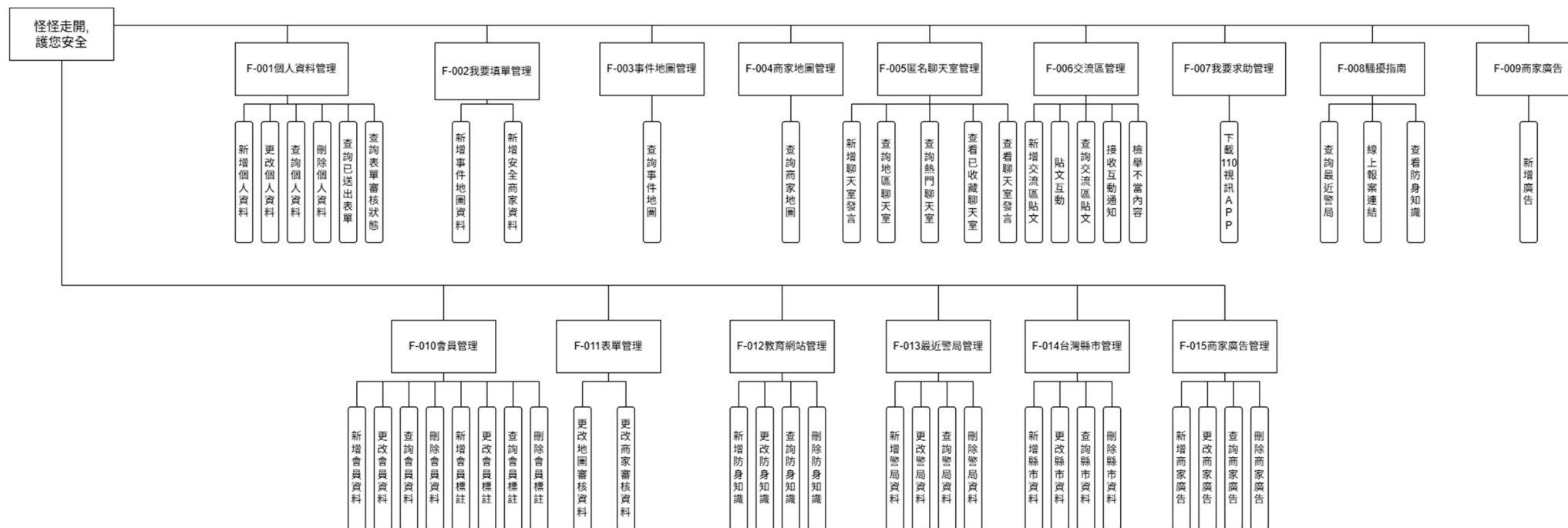
圖 5-1-1 功能分解圖
