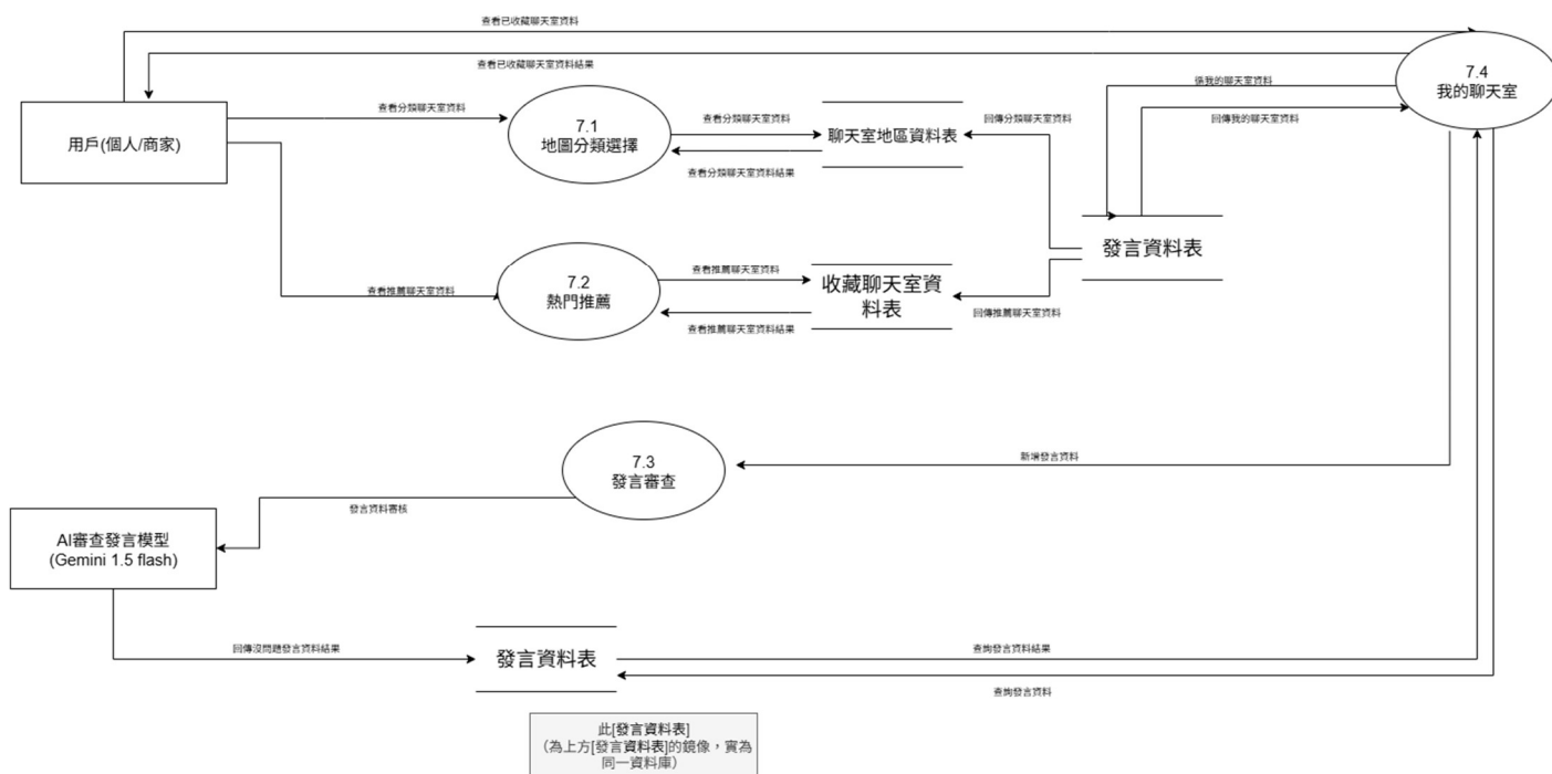
圖 6-1-9 DFD 圖7
