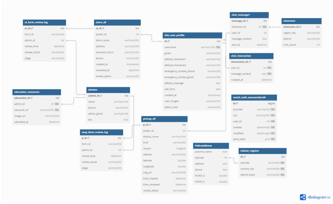
圖 8-1-1 資料庫關聯圖
