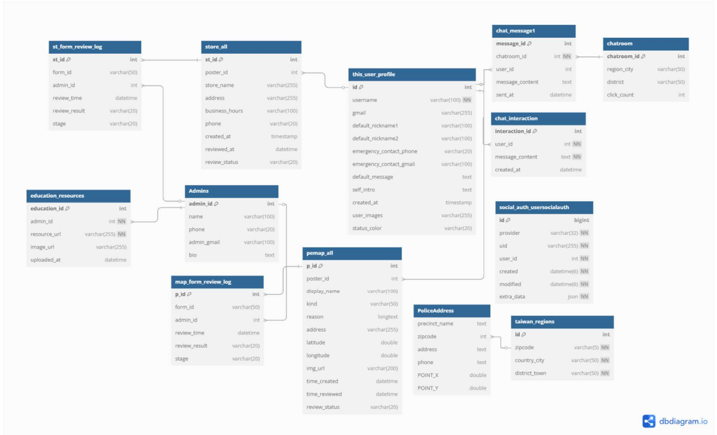
圖 8-1-1 資料庫關聯圖
