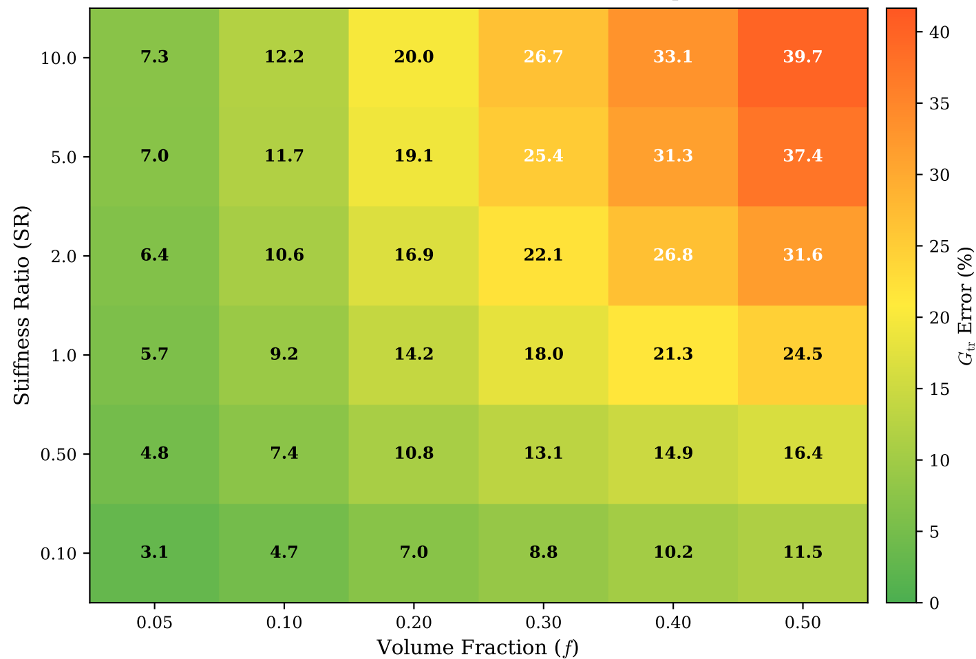
G_{tr} Relative Error (%) — 4-Parameter Isotropic EI Fit
