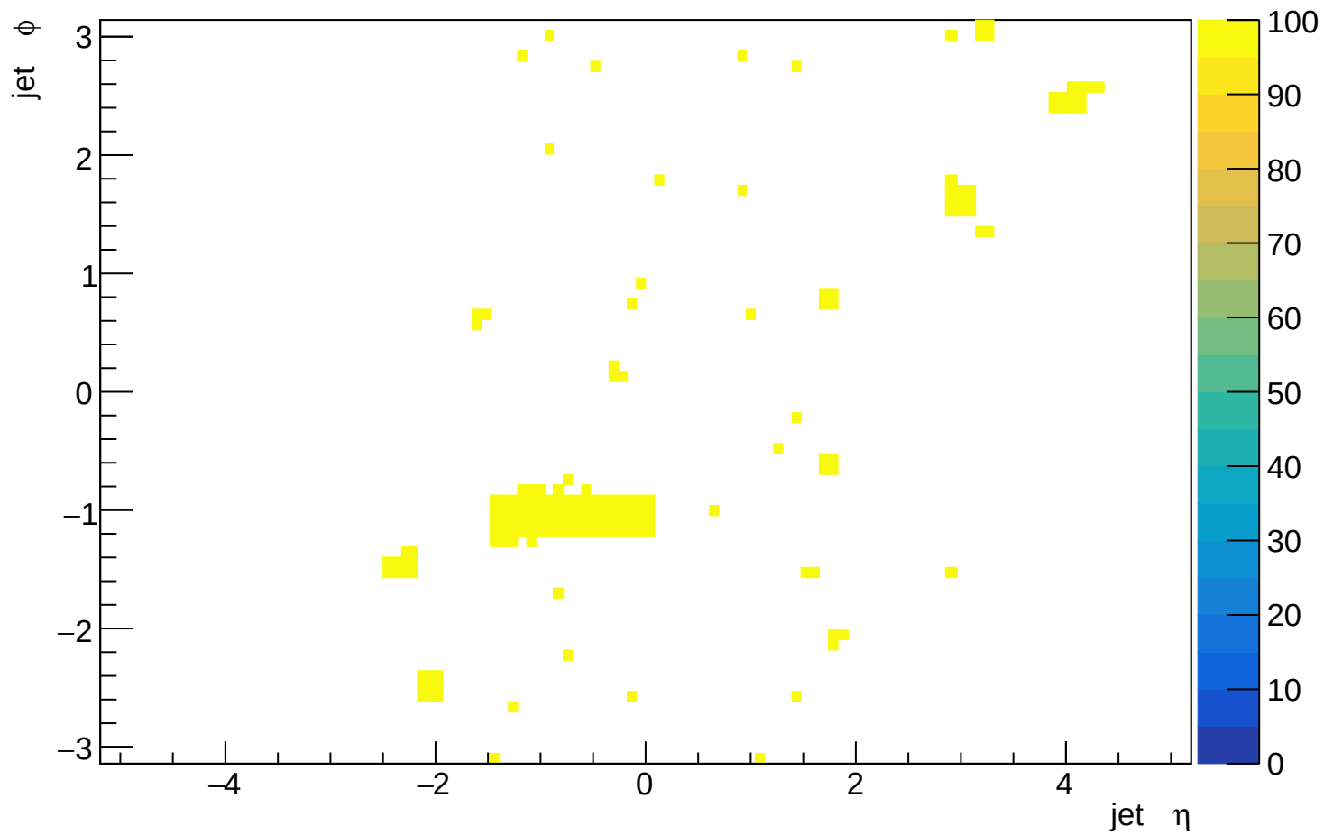
jetvetomap
