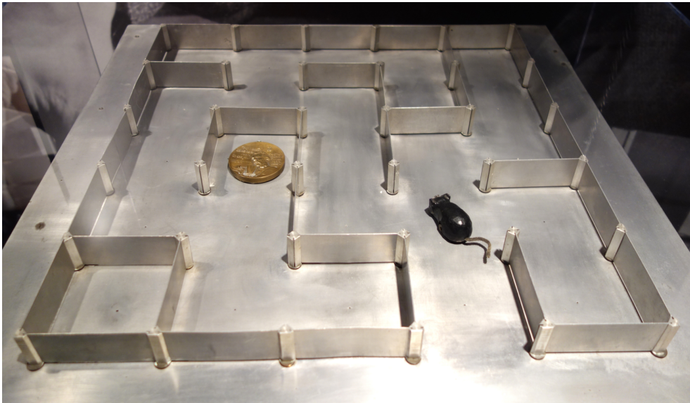
1950 — 새년의 테세우스(MIT Museum 소장). 자석 마우스가 미로를 탐색하다 목표(금색 메달)에 도달하면, 그 경로를 전화 계전기 회로에 저장 — 다음엔 한 번도 틀리지 않고 주파. SNARC와 같은 해, 같은 발상.
