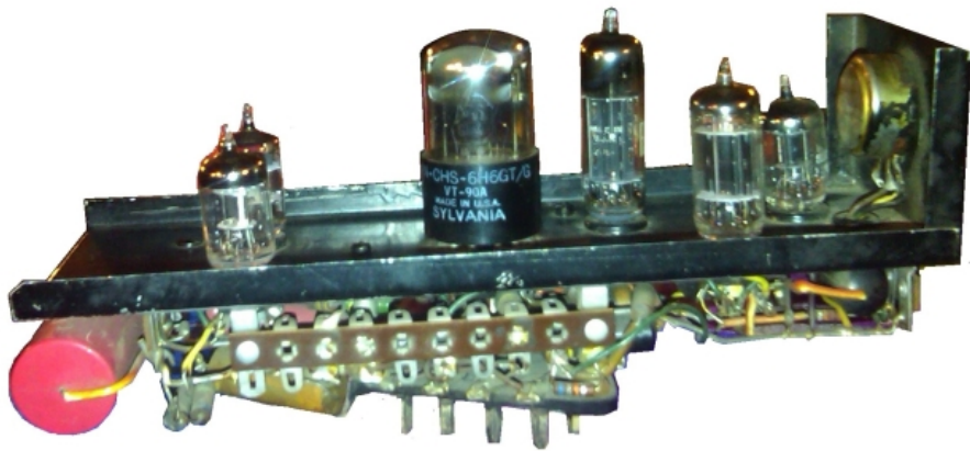
1951 — SNARC의 유일한 현존 부품(“뉴런” 모듈). 진공관 40개로 시냅스 가중치를 흉내낸 최초의 신경망 하드웨어. 민스키가 스키너와 직접 상의해 만든 “스키너식” 보상 기반 학습 회로 — 보상 버튼을 누르면 직전 성공 경로의 시냅스만 강화됨. 1938년 스키너 상자의 원리를 하드웨어로 최초 구현.
