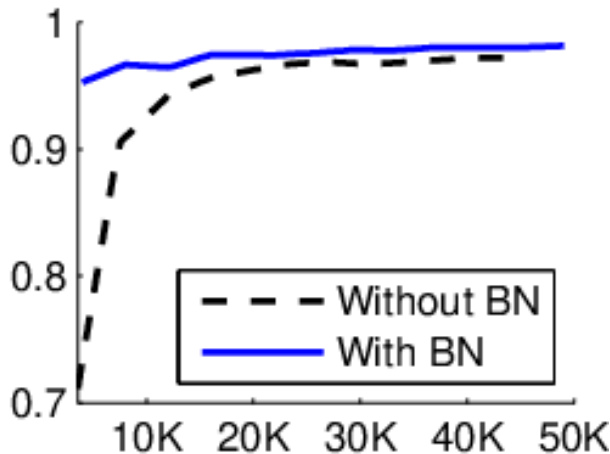
BatchNorm 유무에 따른 MNIST 학습 수렴 속도 (원 논문 Figure 1) — BN이 더 큰 학습률로 적은 스텝에 고 정확도 도달.
