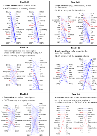
“What Does BERT Look At?” Figure 5 — 특정 헤드들은 인접 토큰, 품사 같은 토큰, 통사 구조적으로 연결된 토큰(주어-동사, 대명사-선행사)에 집중.
