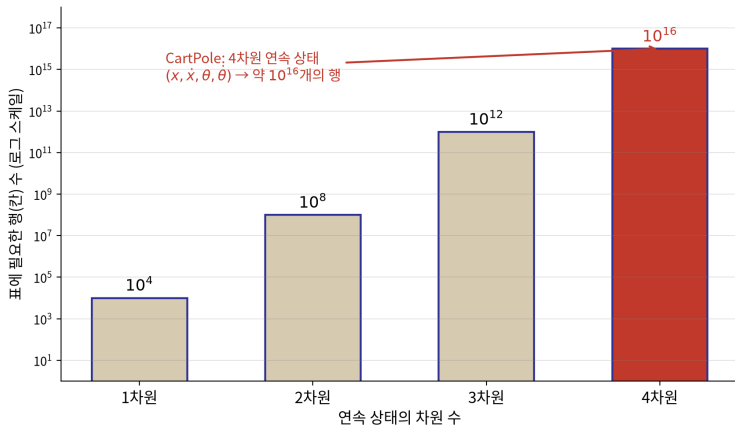
차원의 저주: 0.01 단위로 쪼갠 표 기반 Q-테이블의 크기
