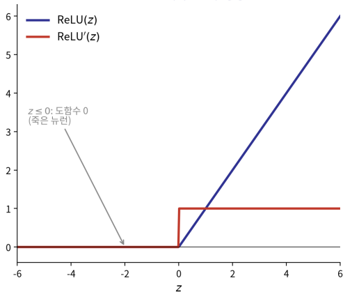
ReLU: z > 0 에서 도함수 항상 1
