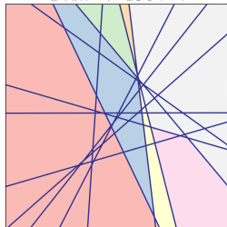
은닉 유닛 12개 → 선형 경계 12개
