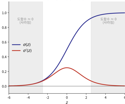
시그모이드: 양 끝에서 그래디언트 소실
