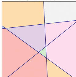
은닉 유닛 4개 → 선형 경계 4개
