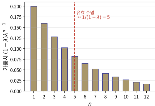
TD( \lambda = 0.8 ): 모든 n 에 기하급수 가중치
