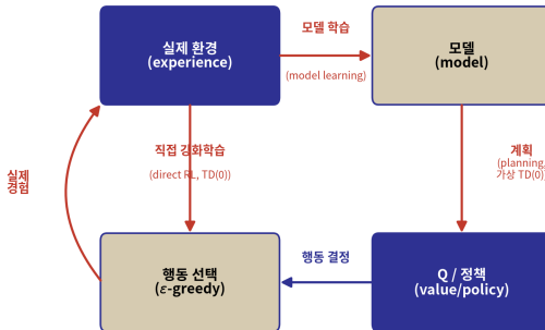
Dyna 아키텍처: 학습과 계획이 하나의 루프로
