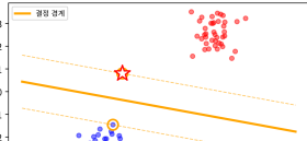
C=1.0: 마진=2.30, n_SV=2, 이상치 y(wTx+b)=+1.00
