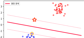
C=100.0: 마진=2.30, n_SV=2, 이상치 y(wTx+b)=+1.00
