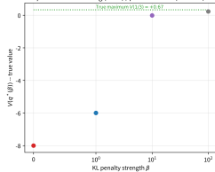
\beta=0 : reward hacking ( V=-8 ) / \beta=100 : frozen ( V=+0.23 )
