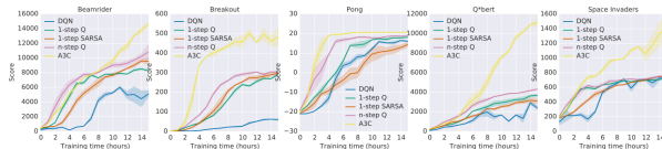
A3C를 포함한 여러 비동기 RL 방법들의 Atari 게임별 학습 곡선 비교 (원 논문 Figure 3).
