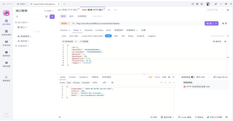
ApiFox 接口测试
