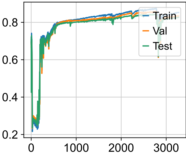
AUC
