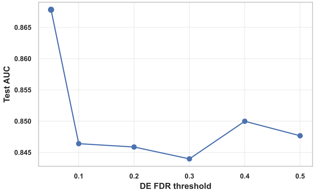
Test AUC Across DE FDR Settings
