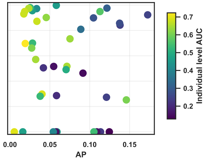
Spectra CD8
