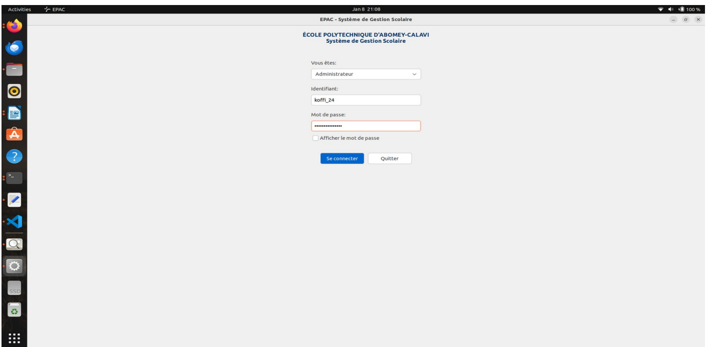
LoginFrame Admin
