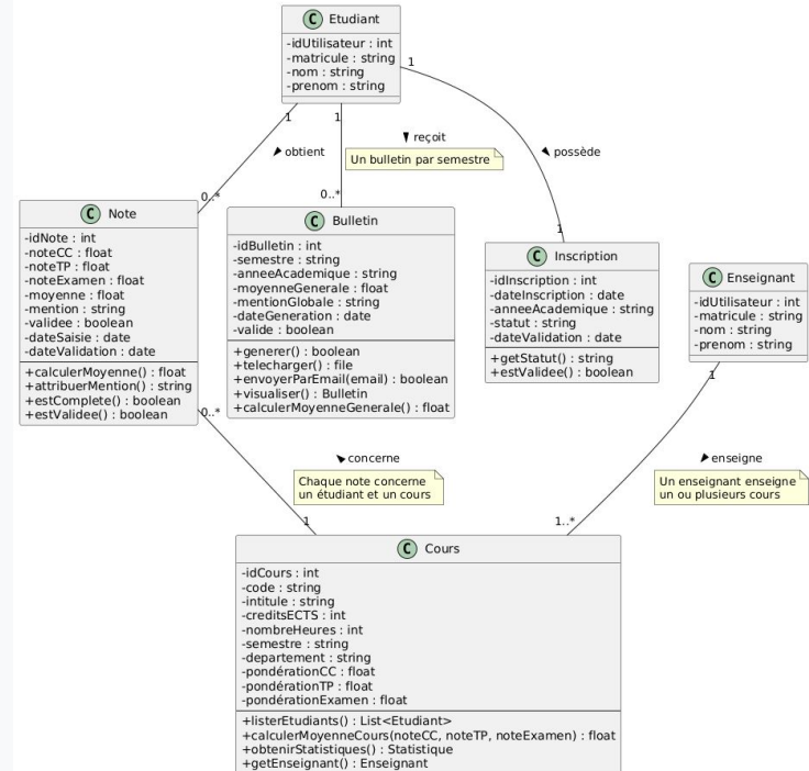
Diagramme de Classes 2/4 - Gestion Académique (Cours, Notes, Bulletin)
