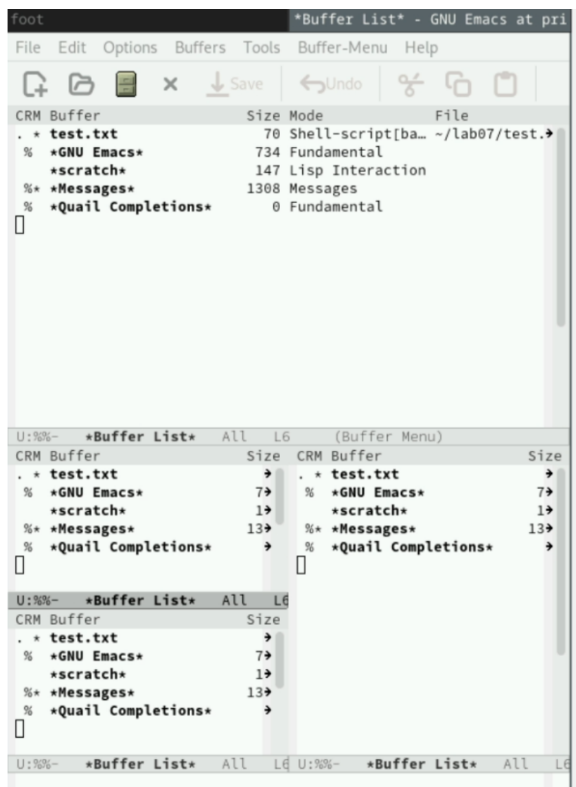
Рис. 3.4: Работа с фреймами в емакс
