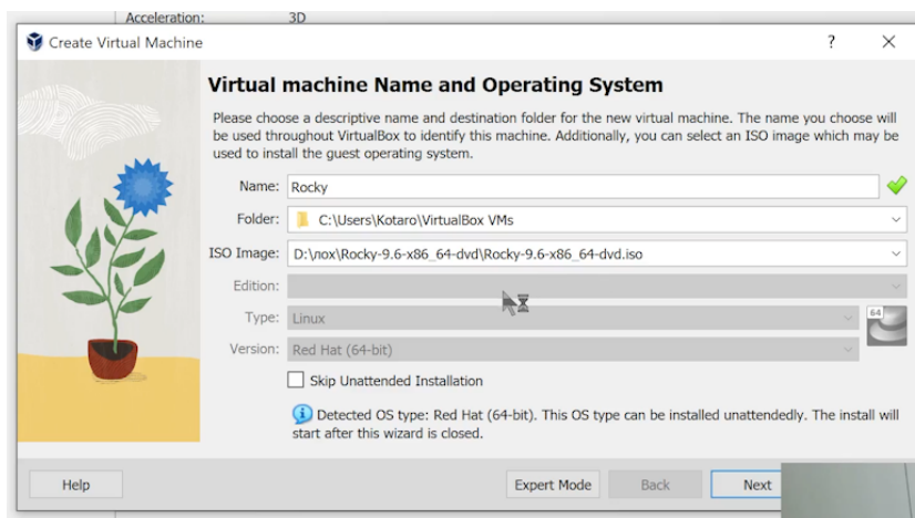
Рис. 3.1: Установочный диск
