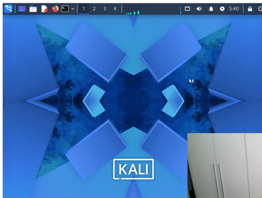
Рис. 3.9: Успешный запуск
