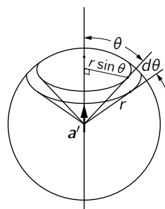
图 32.1: 球截形的 侧面面积为 2\pi r \sin \theta \cdot r d\theta
