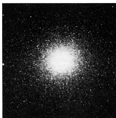
图 7.8: 球状星团
