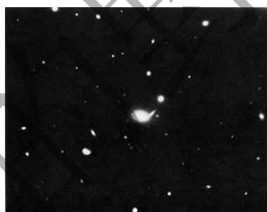
图 7.10: 星系团
