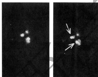
图 7.12: 新星的形成
