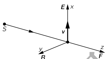
图 34.13: 作用在受电场驱动的电场上的磁力沿着光束方向
