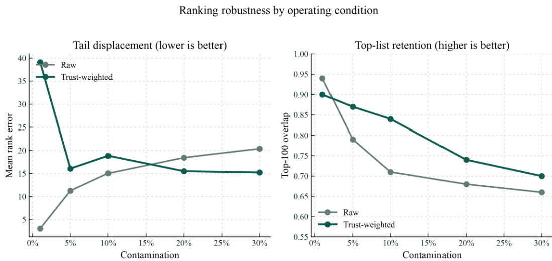
图 A-2 平均排名误差与 Top-100 保留率
