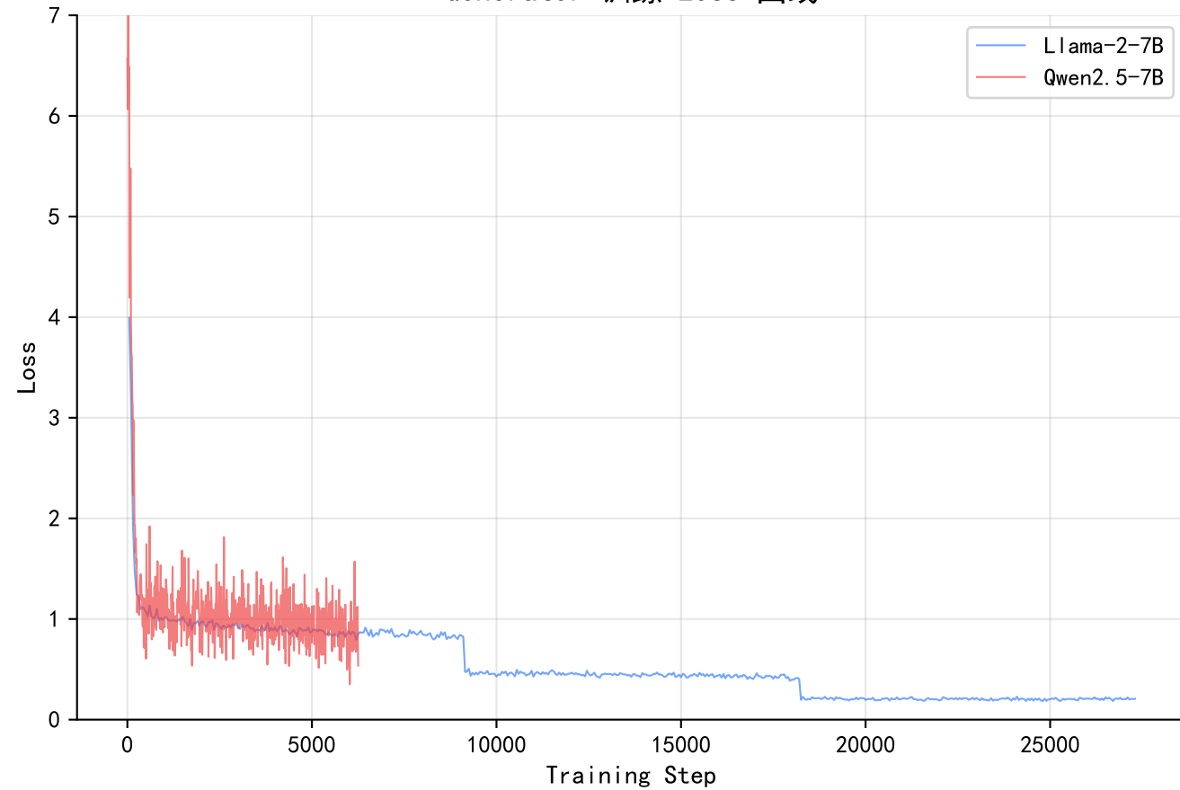
Generator 训练 Loss 曲线
