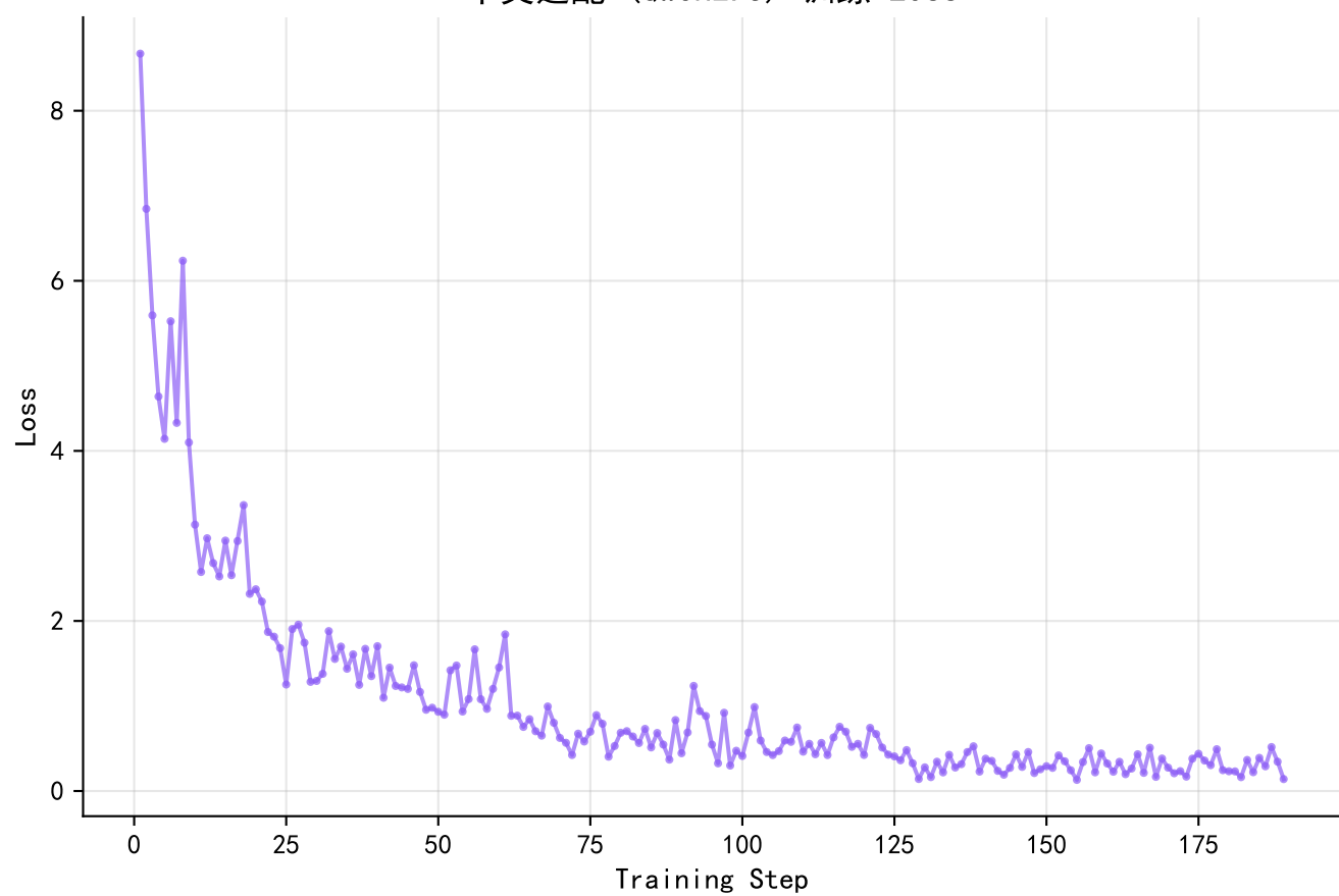
中文适配 (Qwen2.5) 训练 Loss
