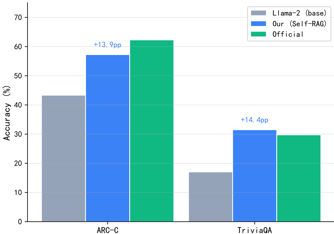
Self-RAG 微调提升幅度 (相对 Llama-2 基线)
