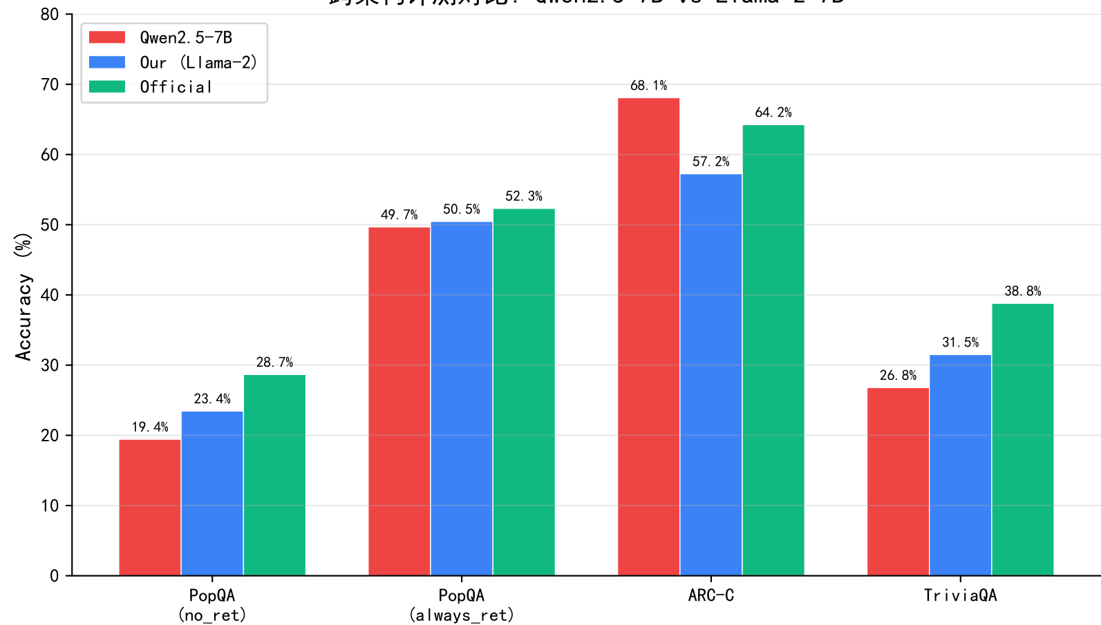
跨架构评测对比: Qwen2.5-7B vs Llama-2-7B
