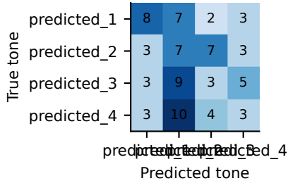
Fusion
