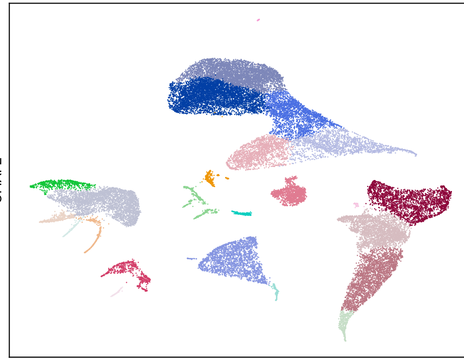
leiden_0.5
