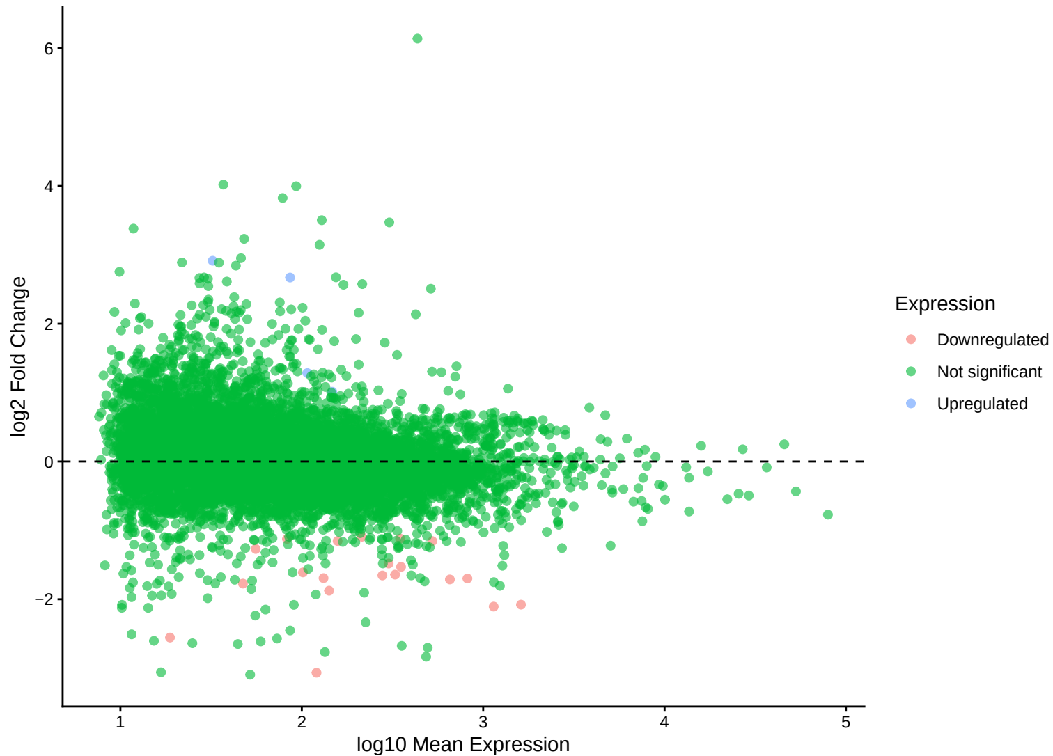
MA Plot: TBT vs DMSO
