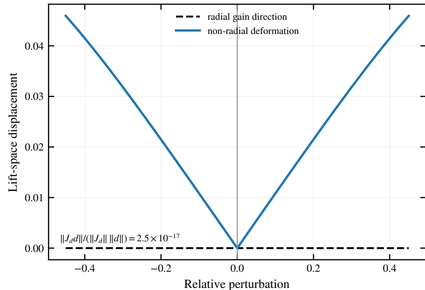
(d) Radial null direction versus deformation
