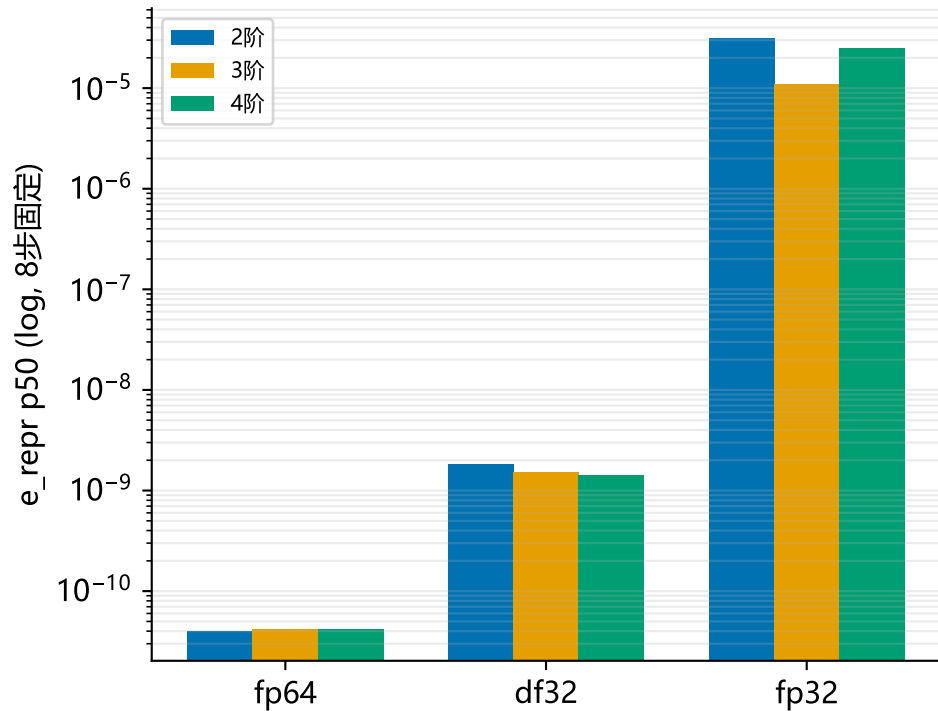
M1-M9 精度:阶次 \uparrow →8步内更准
