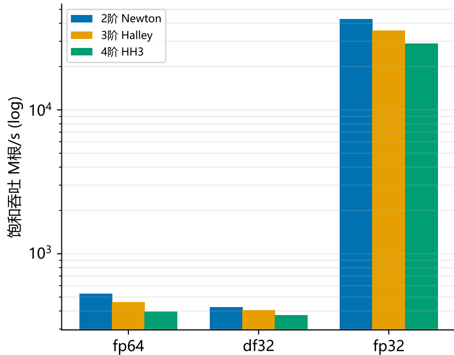
M1-M9 吞吐:阶次 \uparrow →每步更贵吞吐 \downarrow
